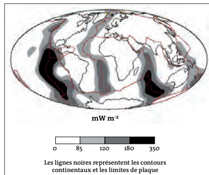
Carte mondiale des flux thermiques exprimés en milliwatts par mètre carré ( \text{mW} \cdot \text{m}^{-2} )
