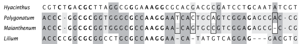
a Séquences partielles obtenues par Mugnier et al. (2000) d'une région non codante de l'ADN ribosomique de 4 plantes précédemment classées dans l'ordre des Liliales (Monocotylédones) et leurs nucléotides communs (identifiées par les bases). A : adénine, T : Thymine, G : Guanine, C : Cytosine. Les tirets indique l'absence de base et les grisés permettent de visualiser les pourcentages de bases communes aux 4 plantes : A 100 %, 75 %, 50 %.
