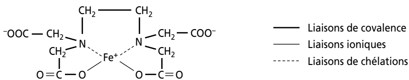
Figure 7.10 - Le chélat de fer EDTA/Fe +++ .
