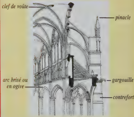
Relevé des éléments les plus représentatifs de l'architecture gothique
