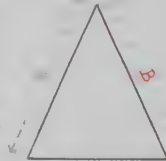
A = B triangle isocèle
