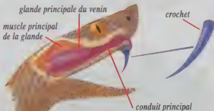
Appareil inoculateur du venin chez une vipère, reconnaissable à sa tête triangulaire.
