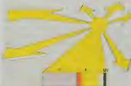
Une radiation est une émission de nature électromagnétique, comme le rayonnement solaire qui est constitué d'ondes électromagnétiques. Ci-dessus, le schéma du spectre solaire : 55% d'infrarouge (IR), 42% de lumière visible (A) et 3% d'ultraviolet (UV).
