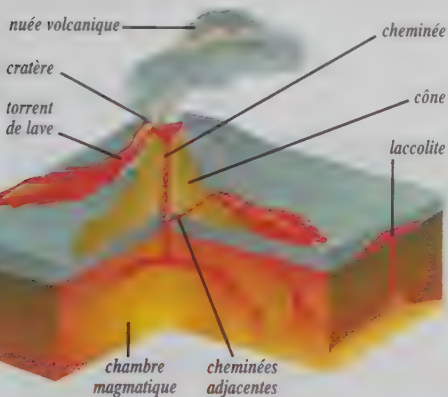
Structure d'un volcan.
