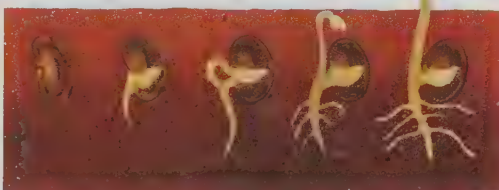
Phases du développement de la graine.
