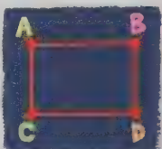
A, B, C et D sont des sommets
