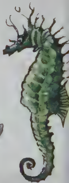
Hippocampe
