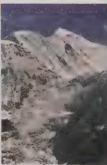
Le glacier montagnard est couvert en surface de cassures béantes, les crevasses.
