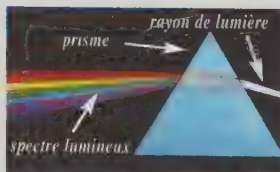
spectre de la lumière
