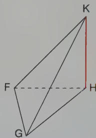
Pyramide dont la hauteur est confondue avec une arête. Base : triangle FGH Hauteur : KH
