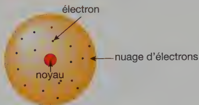
Modèle de l'atome
