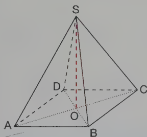
Pyramide régulière à base carrée. Base : carré ABCD de centre O. Axe du carré : (SO) Hauteur : SO
