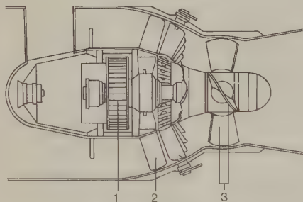
Kaplan à axe horizontal
