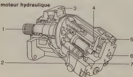
moteur hydraulique
