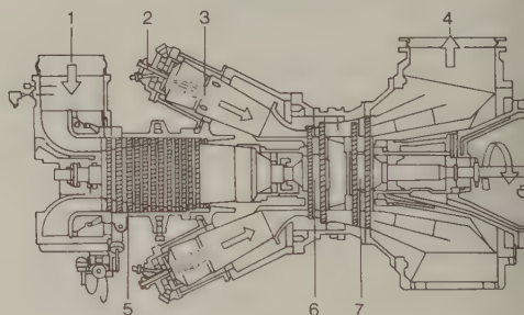
turbine à gaz
