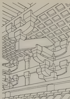
système de consoles en bois supportant une toiture
