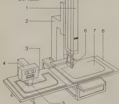
machine de découpage par laser
