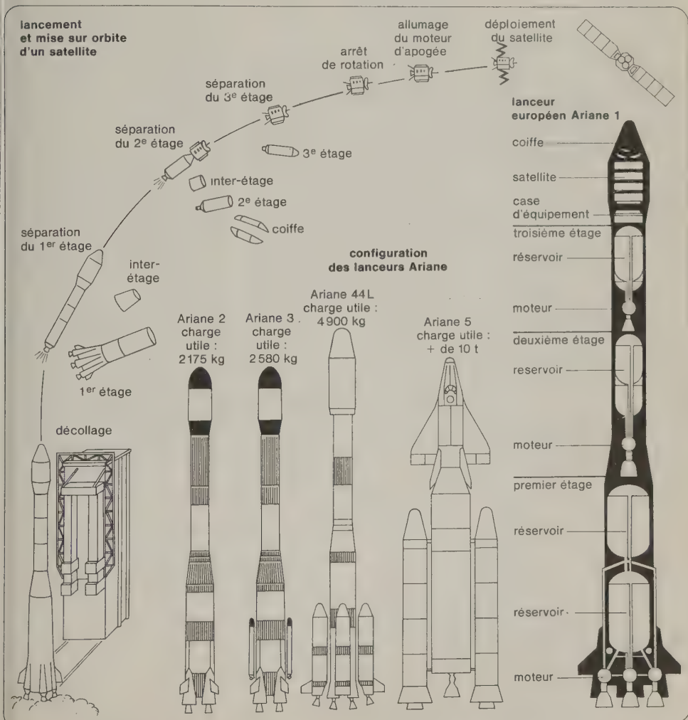
Phases de la mise en orbite d'un satellite, avec la séparation successive des étages de la fusée.
