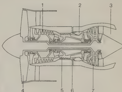
turboréacteur
