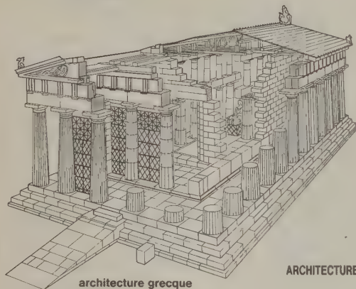
temple dorique d'Athéna Aphaia à Égine (Grèce)
