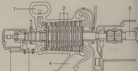
turbine à vapeur
