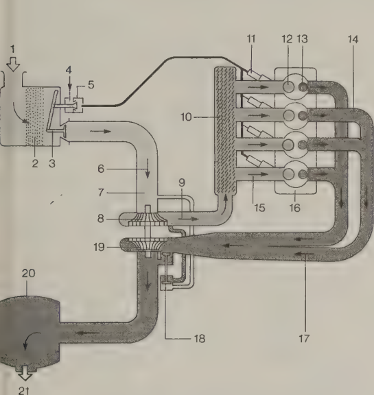
principe de fonctionnement d'un turbocompresseur de suralimentation
