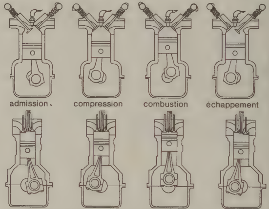
cycle d'un moteur Diesel
