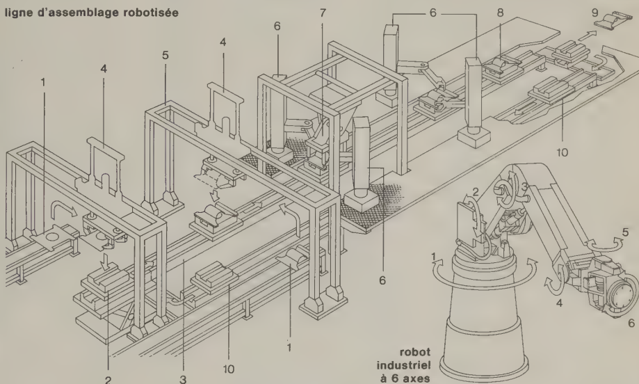
ligne d'assemblage robotisée
