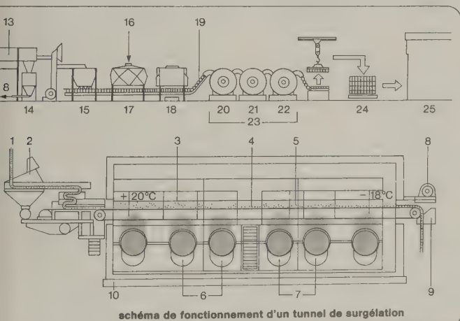
schéma de fonctionnement d'un tunnel de surgélation
