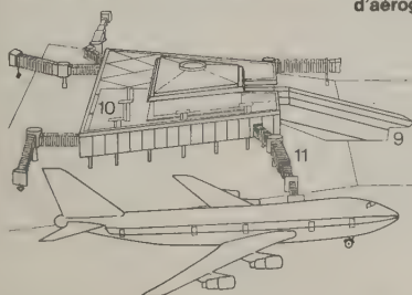
vue en coupe d'un satellite de l'aérogare n° 1 de Roissy
