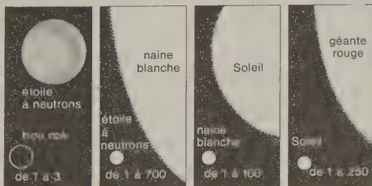
dimensions comparées de diverses étoiles
