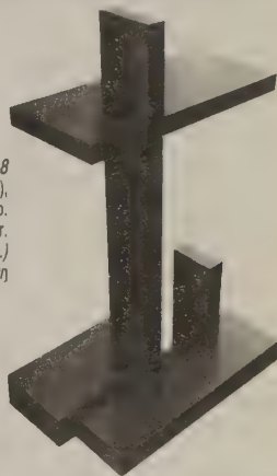
Construction y = ax^2 + bx + 18 (1930), de Georges Vantongerloo. Laiton laqué noir. (Coll. Max Bill, Zurich.) [Doc. Max Bill]
