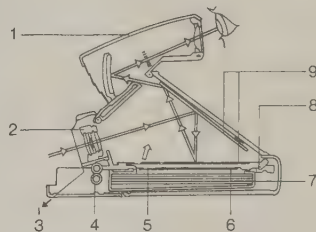
coupe simplifiée d'un appareil reflex Polaroid pour photo instantanée
