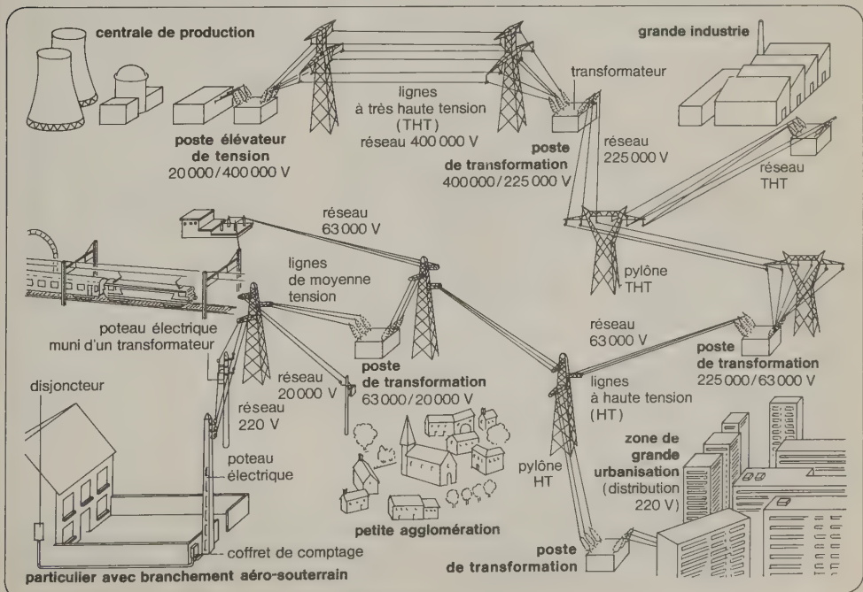
Transport et distribution de l'électricité en France.
