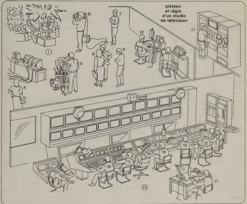
Équipements et personnel d'un studio de télévision.
