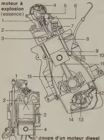
coupe d'un moteur diesel
