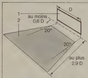
schéma type d'une salle de cinéma, selon la réglementation française
