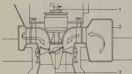
Kaplan à axe vertical
