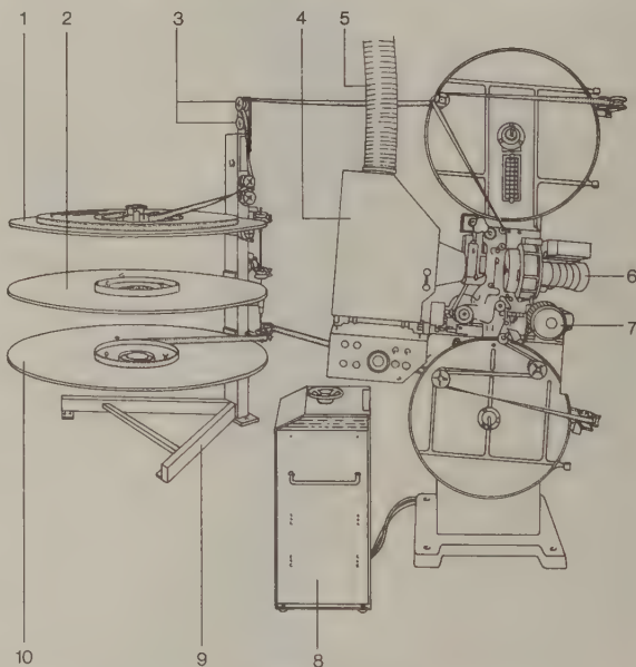
projecteur de cabine équipé d'un dérouleur horizontal à plateau
