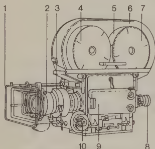
caméra professionnelle de 35 mm
