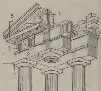
détail de construction d'un temple dorique
