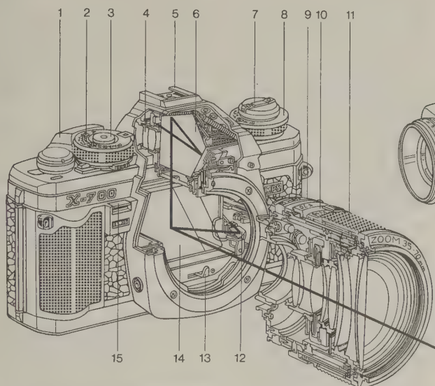
reflex 24x36 avec objectif zoom
