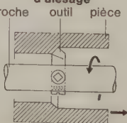
d'alésage
