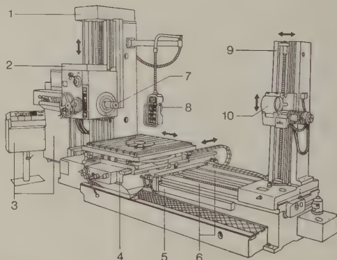
d'alésage
