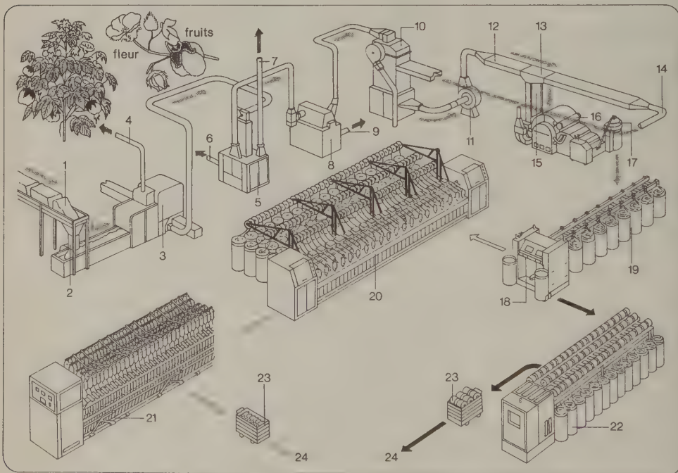
Différentes opérations de la transformation du coton :
