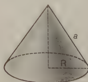
cône de révolution
