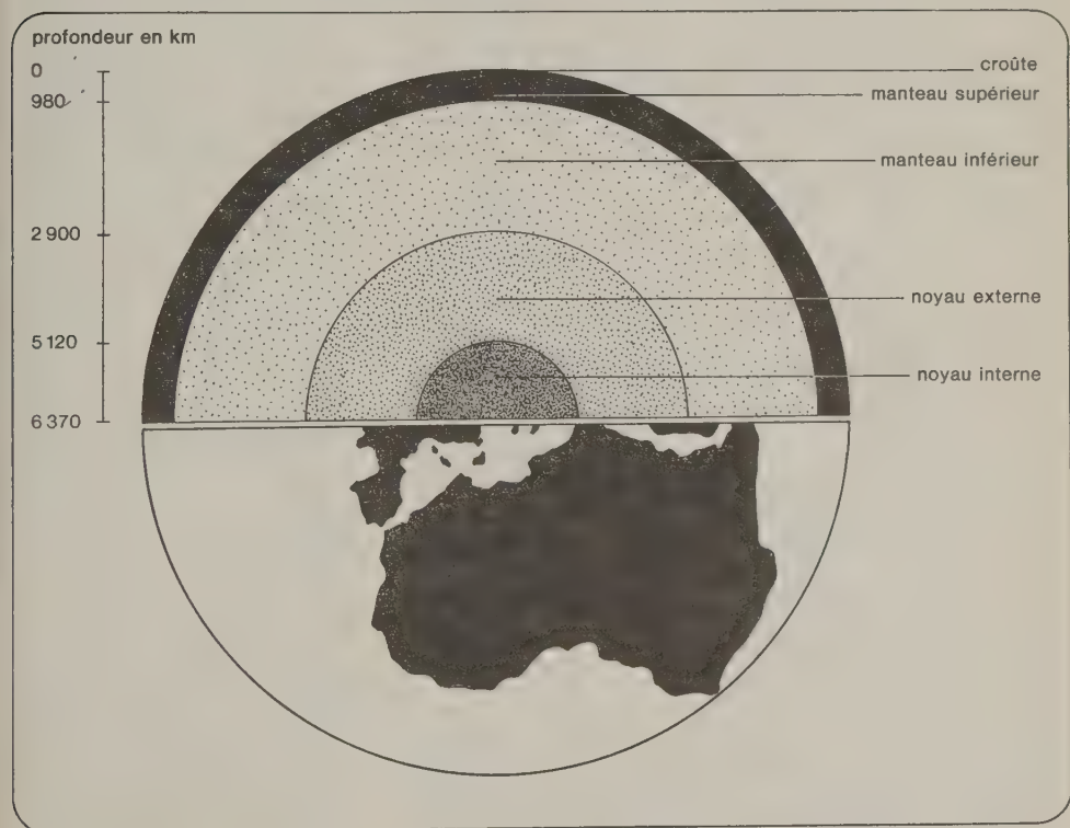
Structure de la Terre.
