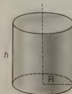
cylindre de révolution
