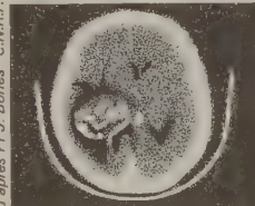
image obtenue par scanner : cerveau avec tumeur
