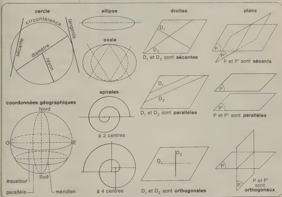
Différentes figures de géométrie et leurs caractéristiques.
