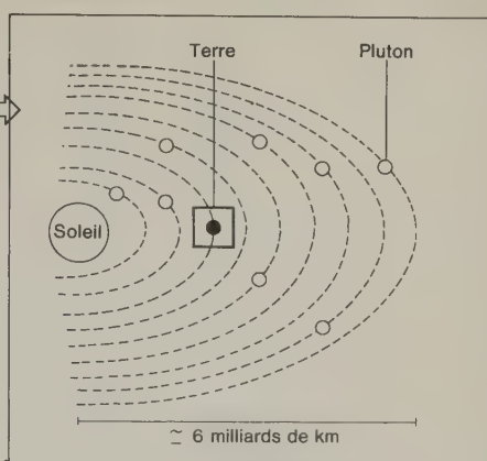
le système solaire
