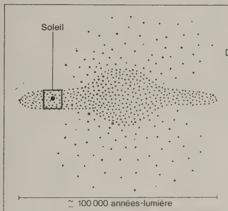
notre Galaxie
