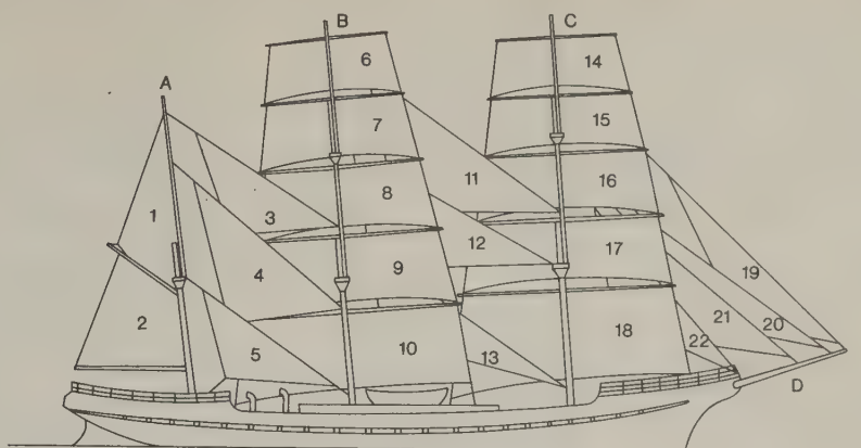
gréements du trois-mâts barque "Belem"
