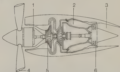
turbopropulseur
