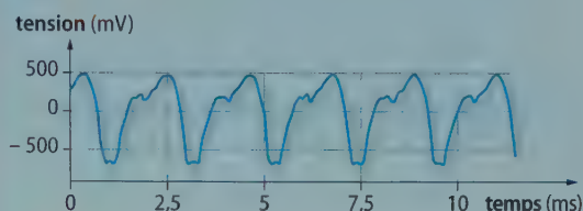
B Enregistrement du son « o » d'une voix féminine
