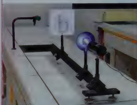
FIG. 10 Image d'un objet par une lentille sur un écran placé de l'autre côté de la lentille.
