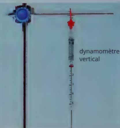
FIG. 2 La valeur de la force se mesure avec un dynamomètre.
