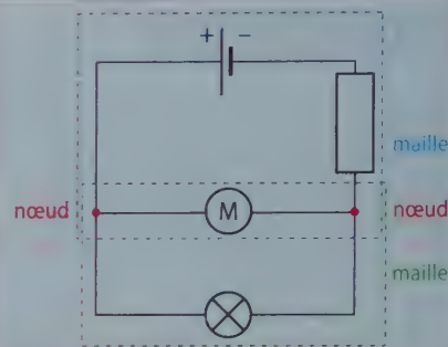
FIG. 2 Schéma normalisé du circuit électrique de la figure 1.
