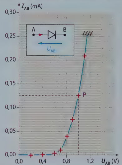
FIG. 6 Caractéristique tension-intensité d'une diode : I_{AB} = g(U_{AB}) .
