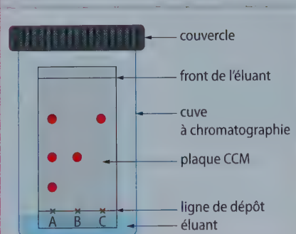
FIG. 6 Sur le chromatogramme apparaissent à des hauteurs différentes les divers constituants du mélange, identifiés par comparaison avec des échantillons témoins.
