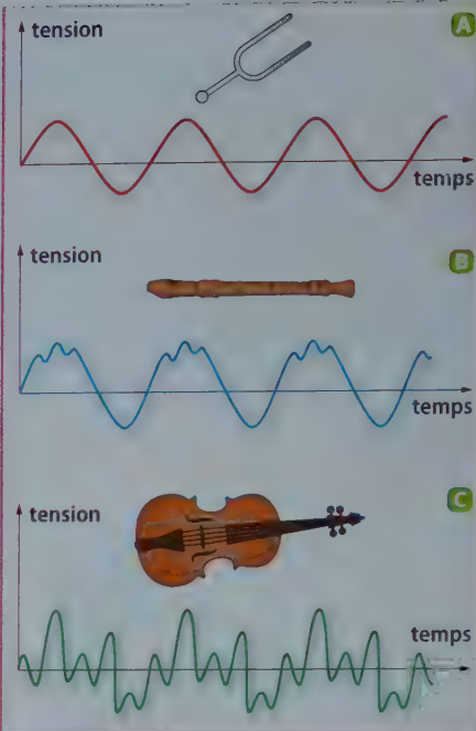
FIG. 7 Une même note jouée par trois instruments de musique différents.
