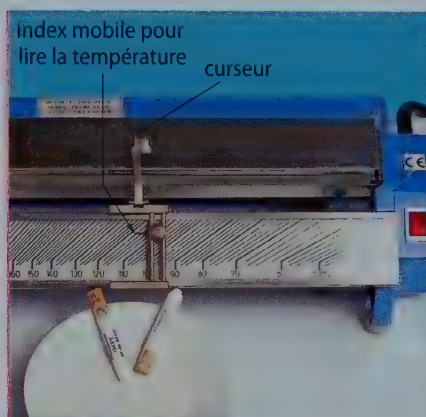
FIG. 5 Détermination de la température de fusion à l'aide d'un banc Kofler. Le solide est déplacé progressivement à partir du point le moins chaud jusqu'au point de la plaque où il commence à fondre ( FICHE PRATIQUE ➔ p. 304).
