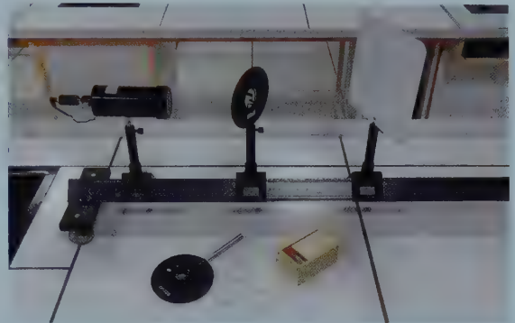
Le dispositif expérimental : un banc optique.
