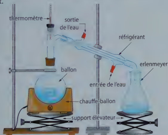
Montage de distillation
