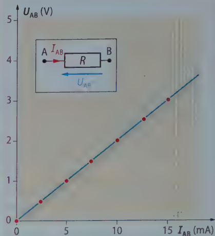
FIG. 8 Caractéristique intensité-tension d'un conducteur ohmique : U_{AB} = f(I_{AB}) .
