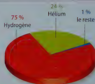
FIG. 1 Les éléments hydrogène et hélium sont les plus abondants dans l'univers.
