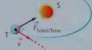
FIG. 3 L'action mécanique qu'exerce le Soleil sur la Terre modifie la trajectoire rectiligne que la Terre tendrait à suivre en l'absence d'actions.
