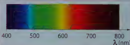
FIG. 3 Le domaine du visible couvre les radiations de longueur d'onde entre 400 et 800 nm.
