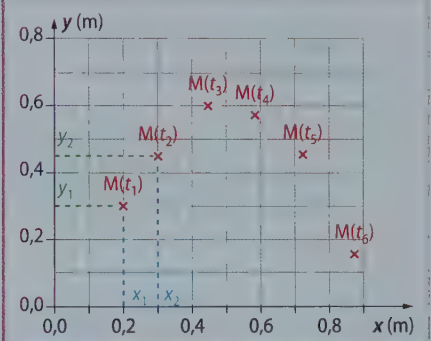
FIG. 4 Le point matériel M est repéré par ses coordonnées x et y à différents instants t .
