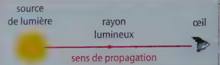
FIG. 1 Trajet d'un rayon lumineux jusqu'à un observateur.
