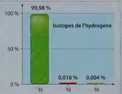
FIG. 3 L'hydrogène existe sous la forme de trois isotopes stables : l'isotope le plus abondant ^1\text{H} , et deux isotopes plus lourds, le deutérium ^2\text{H} et le tritium ^3\text{H} .
