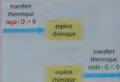
FIG. 1 Convention de signes du transfert thermique Q .
