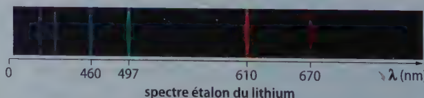
spectre étalon du lithium
