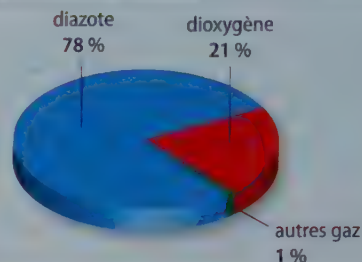
FIG. 2 Composition volumique de l'air.
