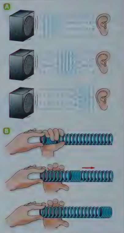
FIG. 2 La propagation d'un signal sonore dans l'air A est analogue à la propagation d'une déformation dans un ressort B .
