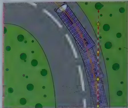
FIG. 1 Trajectoire d'un bus et mouvement de son passager sans ceinture de sécurité.
