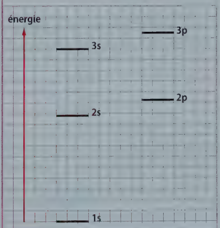
FIG. 4 Énergie des sous-couches électroniques.
