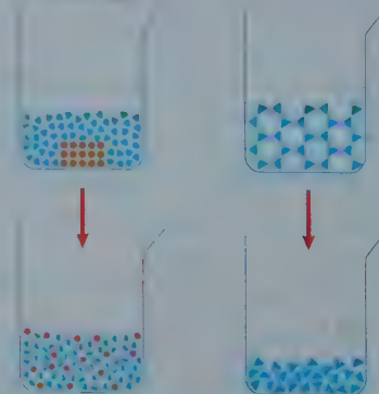
FIG. 3 Comportement microscopique des particules de matière.
