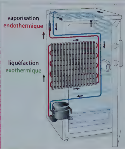
FIG. 5 Fonctionnement d'un réfrigérateur.
