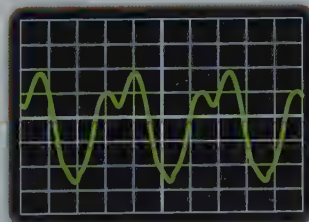
A Enregistrement du son de la guitare base de temps : 2 \text{ ms} \cdot \text{div}^{-1} sensibilité verticale : 200 \text{ mV} \cdot \text{div}^{-1}
