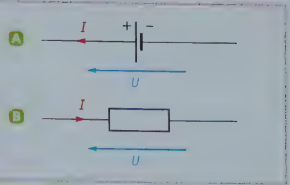
FIG. 5 Convention générateur A et convention récepteur B.
