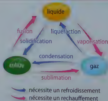
FIG. 3 Les changements d'état.
