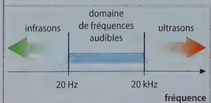
FIG. 6 Domaines de fréquences des sons chez l'humain.
