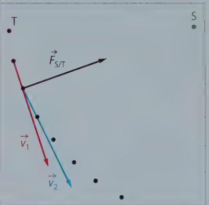
FIG. 5 Variation du vecteur vitesse \vec{v} de la Terre entre deux instants successifs.
