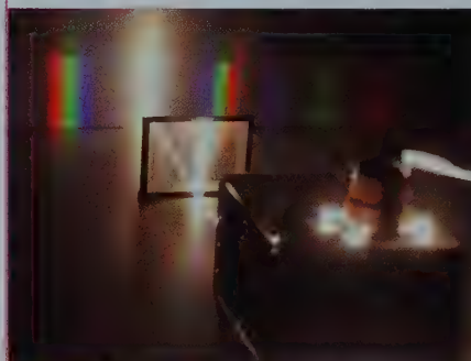
FIG. 6 Dispersion de la lumière blanche par un réseau (un ensemble de traits serrés) : les spectres obtenus révèlent toutes les couleurs de l'arc-en-ciel.
