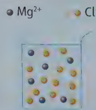
FIG. 4 Schématisation du chlorure de magnésium en solution.
