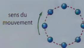
B Mouvement circulaire uniforme
