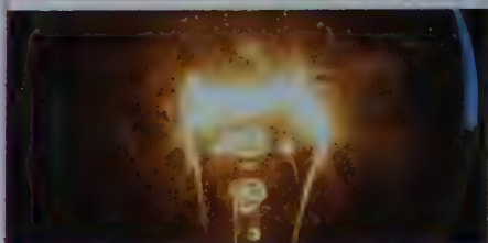
FIG. 8 Un filament chauffé passe du rouge au blanc au fur et à mesure que la température augmente.
