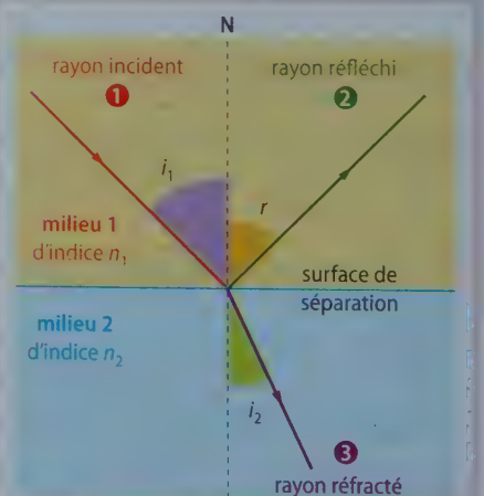
FIG. 4 Réflexion et réfraction d'un rayon à la surface de séparation entre deux milieux.
