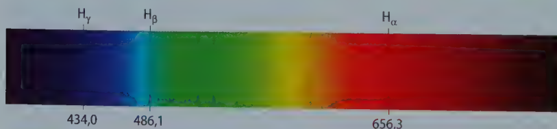
FIG. 11 Spectre du Soleil. Trois raies noires caractéristiques de l'hydrogène y sont repérées : l'atmosphère du Soleil comporte en effet de l'hydrogène.
