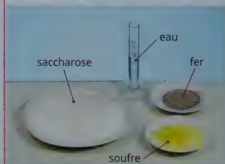
FIG. 6 Quatre échantillons d'eau, de saccharose, de fer et de soufre contenant chacun une mole d'entités chimiques.
