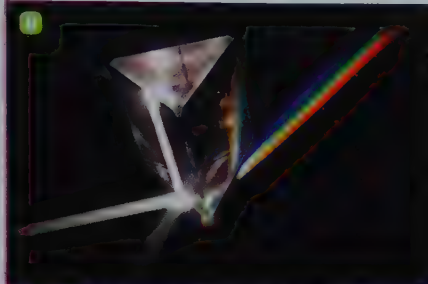
FIG. 5 Le spectre de la lumière blanche est visible sur un CD A et à la sortie d'un prisme B, deux systèmes dispersifs.
