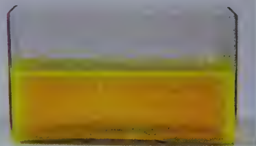
FIG. 5 Réflexion et réfraction de la lumière au passage de l'air à l'eau.
