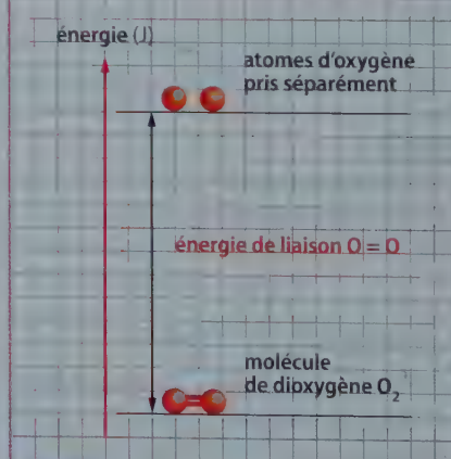
FIG. 7 Énergie de la liaison O=O dans la molécule de dioxygène O 2 .
