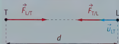
FIG. 4 Interaction gravitationnelle entre la Terre T et la Lune L.
