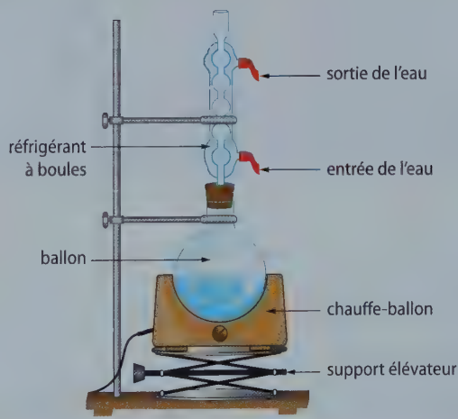
Montage de chauffage à reflux
