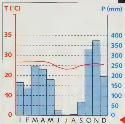
Diagramme climatique de Lambaréné (Gabon)
