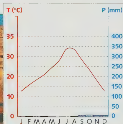
Diagramme climatique de Tindouf (Algérie)
