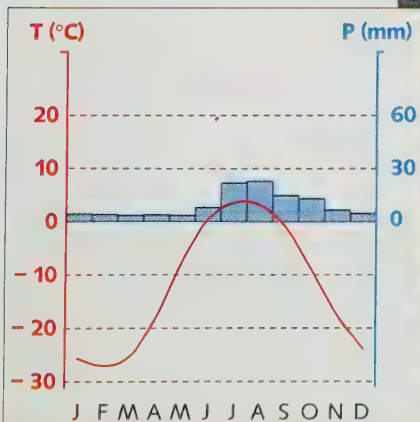
Diagramme climatique de Barrow (Alaska)
