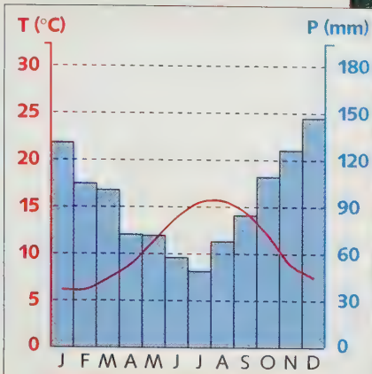
Diagramme climatique de Brest
