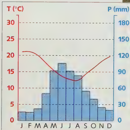
Diagramme climatique du Cap
