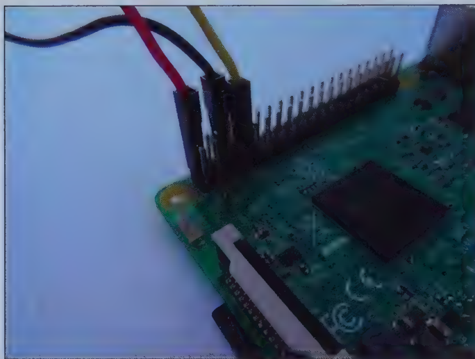
Figure 16.7 : Les trois straps branchés sur le GPIO.
