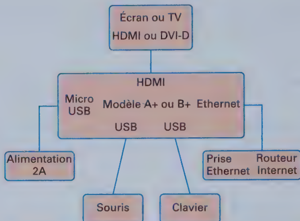
Figure 1.4 : Branchements d'un Raspberry sans concentrateur USB.
