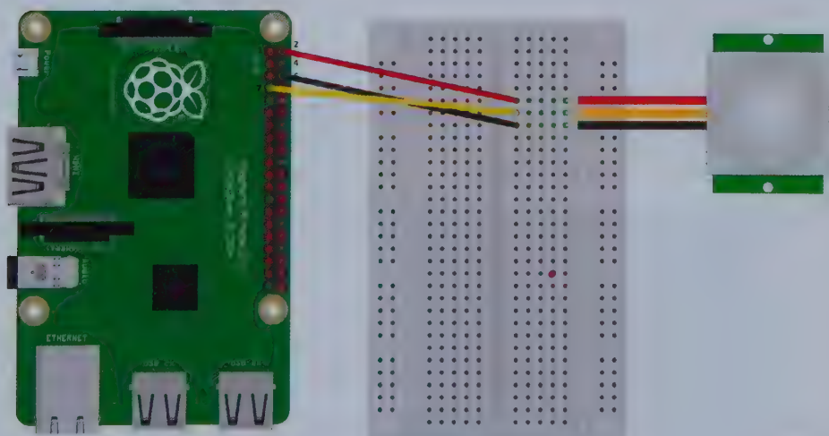
Figure 16.6 : Schéma de branchement sur le GPIO.
