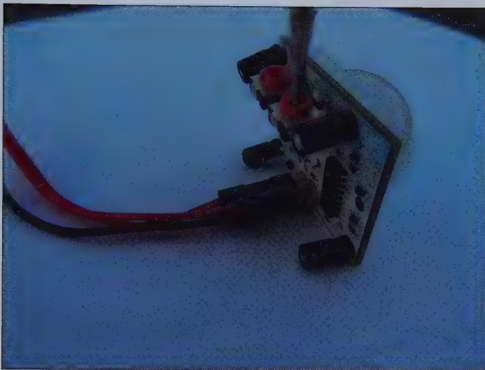
Figure 16.11 : Réglage du seuil de détection avec un tournevis.
