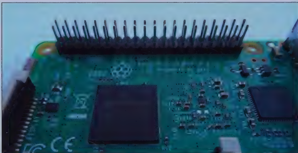
Figure 16.1 : Vue générale du connecteur GPIO.
