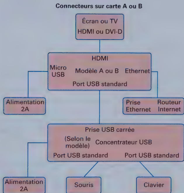
Figure 1.3 : Branchements d'un Raspberry avec concentrateur USB.
