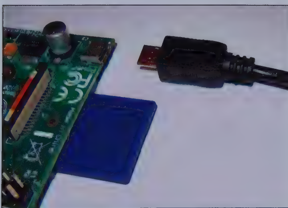
Figure 3.7 : Insertion du câble micro USB d'alimentation.
