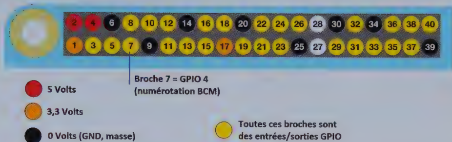
Figure 16.3 : Schéma du connecteur GPIO.
