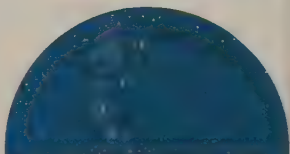
en janvier vers 22 h 00
