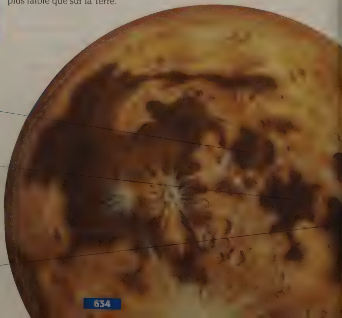
mer de la Sérénité
