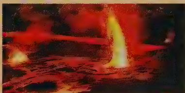
▲ Vue d'artiste de la Terre, il y a 4,5 milliards d'années.
