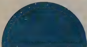
en septembre vers 22 h 00
