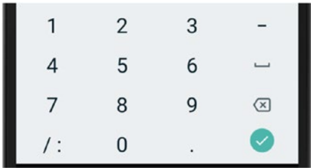
Figure 4-6. TextInputType.datetime
