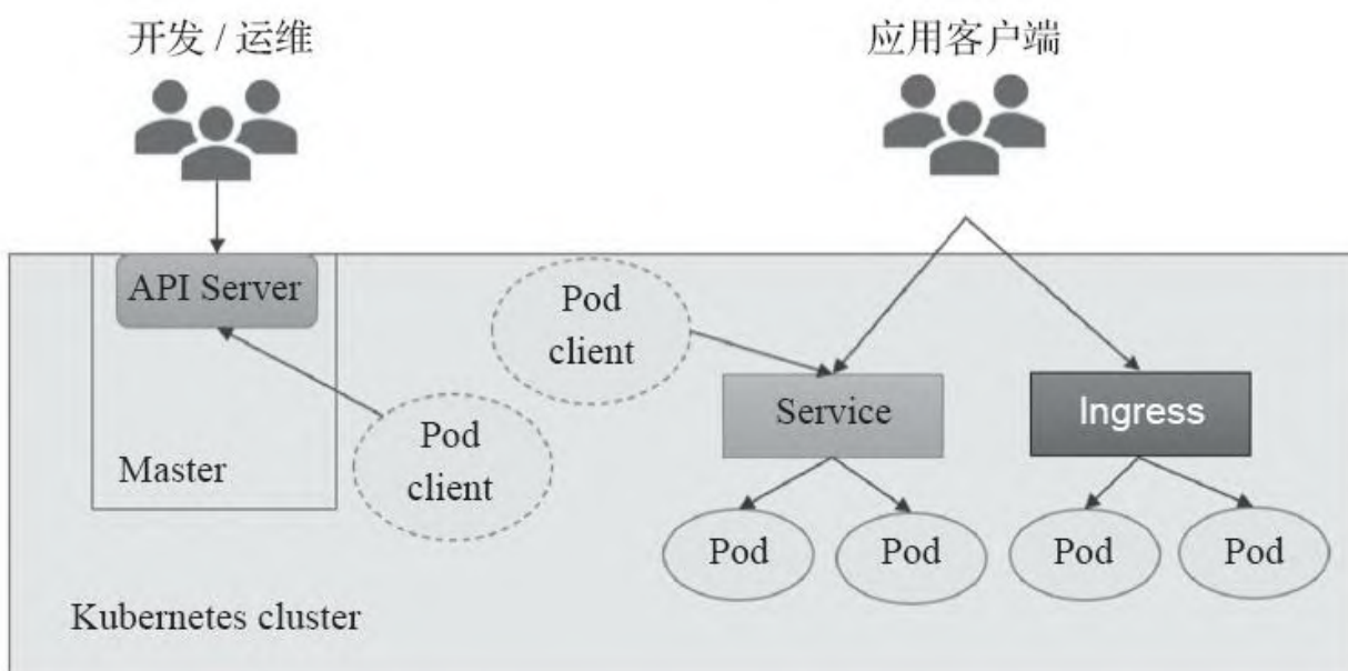
图1-14 Kubernetes客户端及其类型
