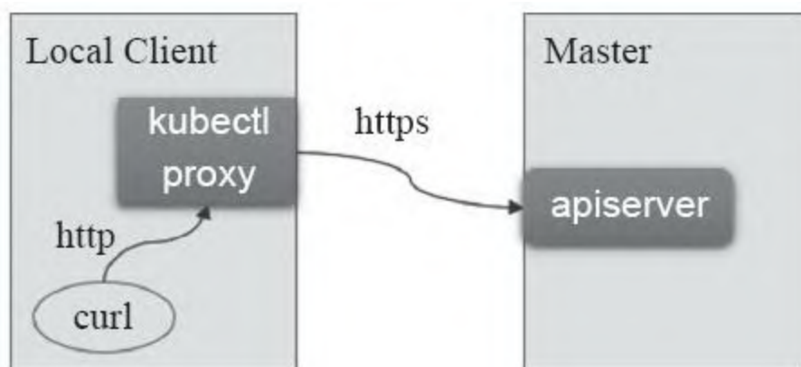
图3-3 kubectl在本地代理API Server
