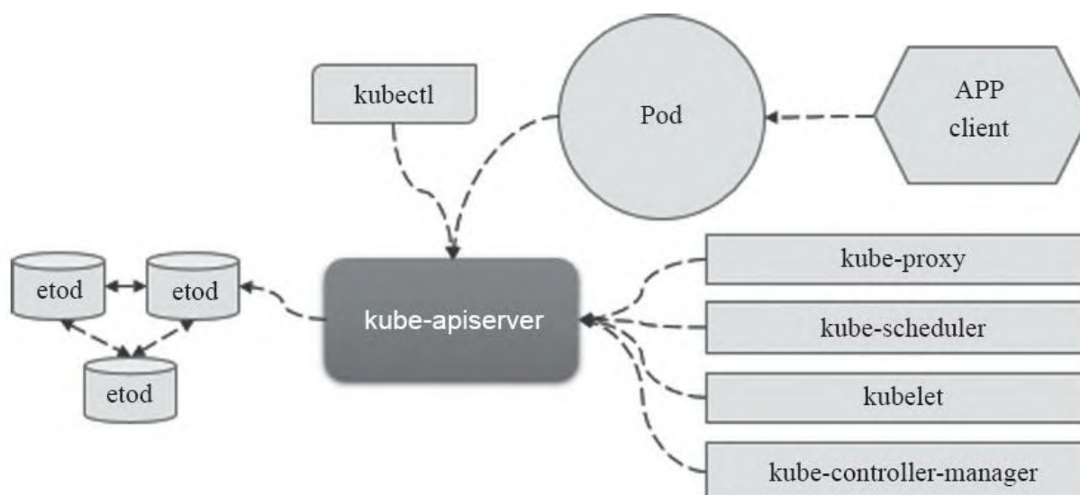
图10-4 Kubernetes的SSL/TLS通信
