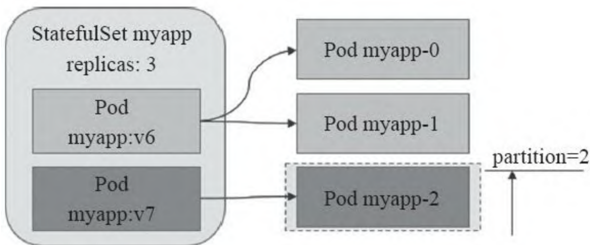
图9-5 金丝雀发布
