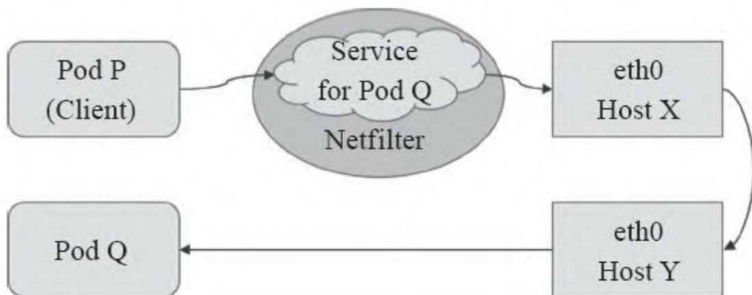
图11-4 Service和Pod
