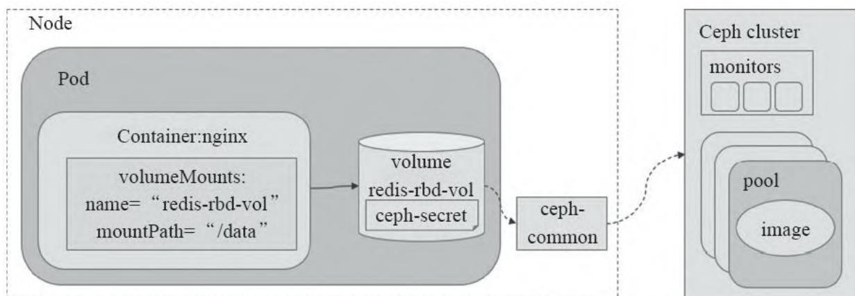
图7-3 RBD存储卷
