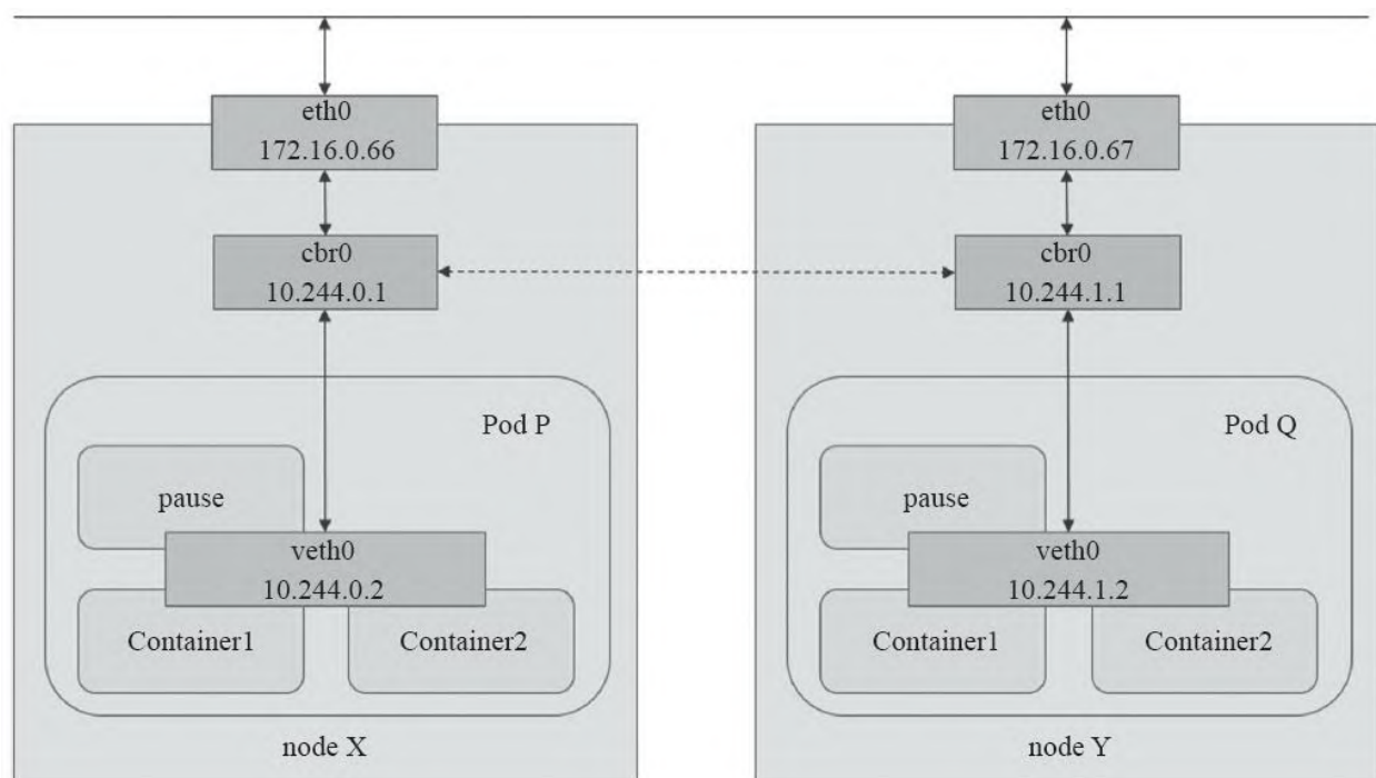
图11-3 Pod网络
