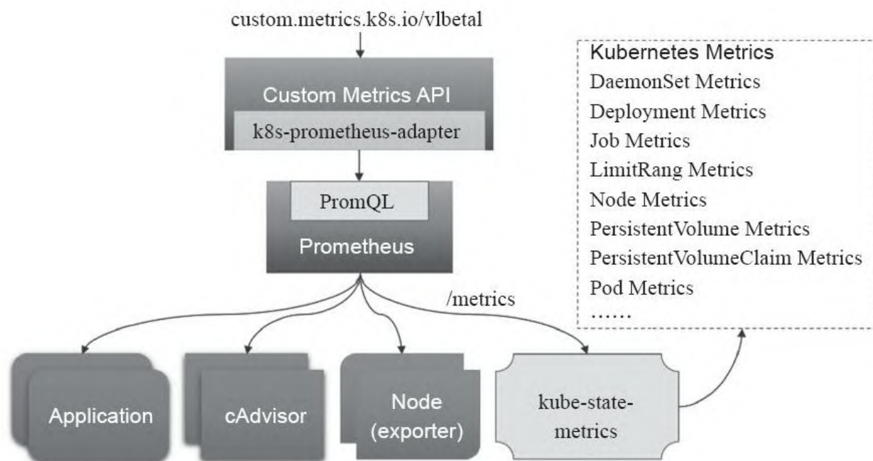
图14-7 自定义指标
