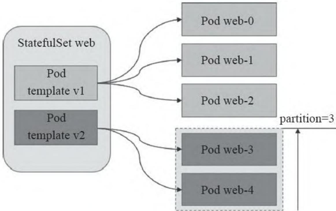
图9-3 ReplicaSet分区滚动更新
