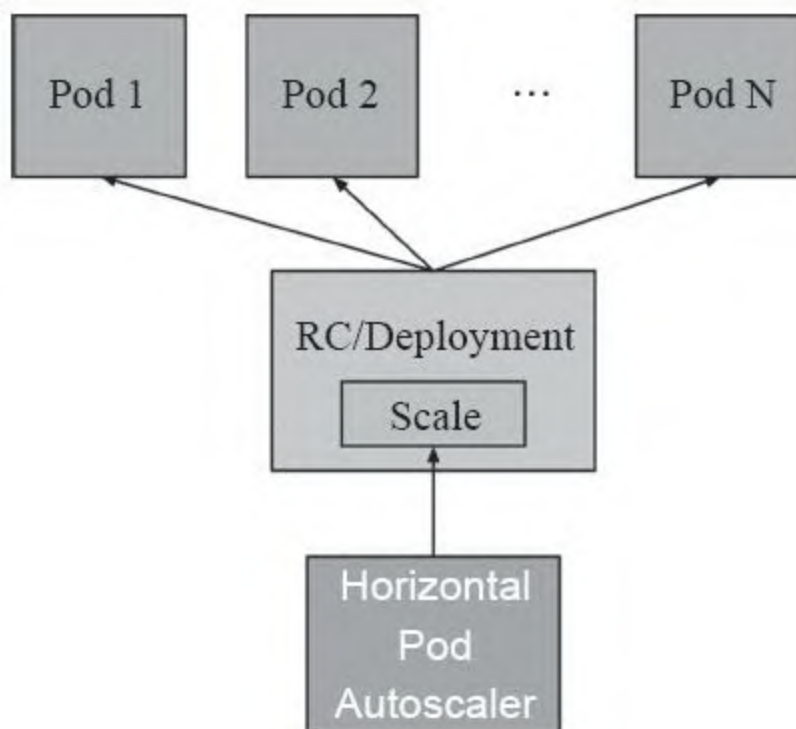
图14-12 HPA控制器示意图
