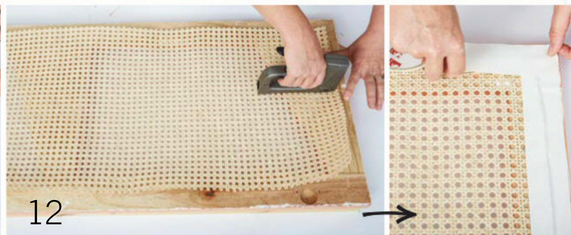
12 Kram die rottangmat vas; trek dit styf terwyl jy werk. Plak hegband oor die mat se rande om dit netjies te hou.
