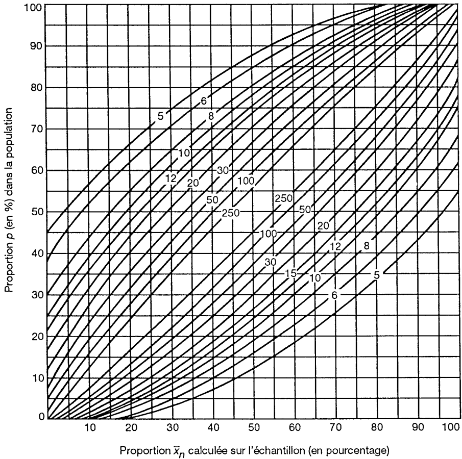
Abaque 1 Intervalles de confiance pour une proportion p Intervalle bilatéral de niveau de confiance 0,90 Intervalles unilatéraux de niveau de confiance 0,95
