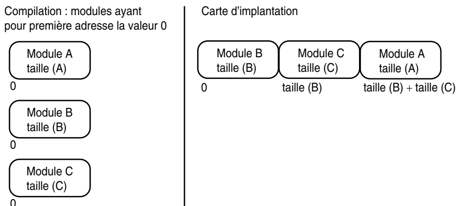
Figure 3.7 Carte d'implantation.
