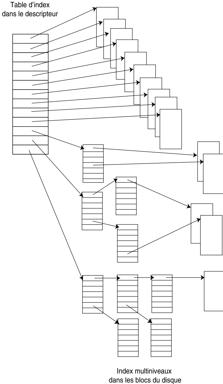
Figure 14.9 Index dans le système Unix.
