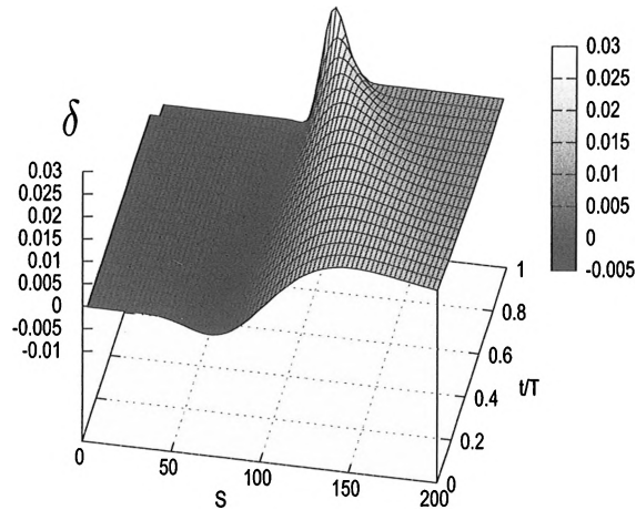
Figure 7.7 - Le « delta », en fonction du prix du stock S et du temps t , pour E = 100 , r = 6\% , \sigma = 0.3 .
