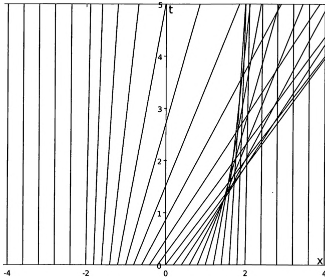
Figure 7.5 – Les caractéristiques de l'équation de Burgers dans le cas où \mu_0(x) = e^{-x^2}
