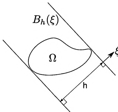
Figure D.3 - Domaine inclus dans une bande
