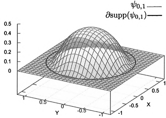
Figure 4.2 - \psi_{0,1} sur \mathbb{R}^2
