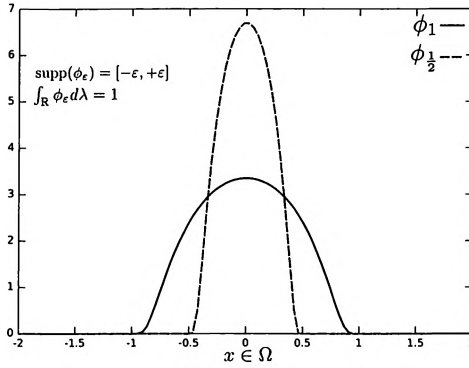
Figure 4.3 – Éléments d'une approximation de l'identité
