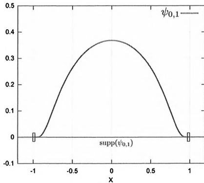
Figure 4.1 - \psi_{0,1} sur \mathbb{R}
