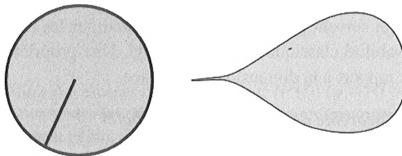
Figure D.2 - Exemples de domaines non-réguliers
