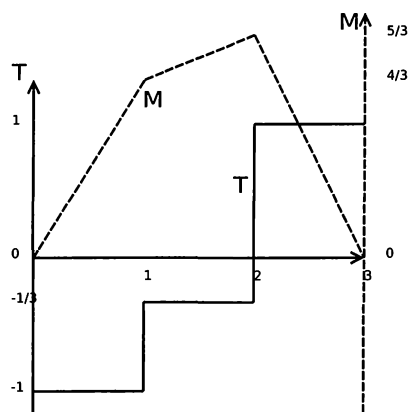
Figure 4.5 - Effort et moment le long de la poutre
