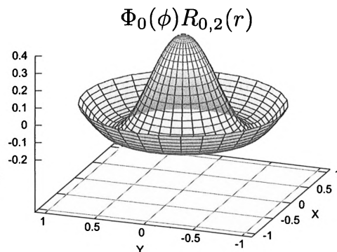
Figure 6.4 - Mode(0,2) du tambour
