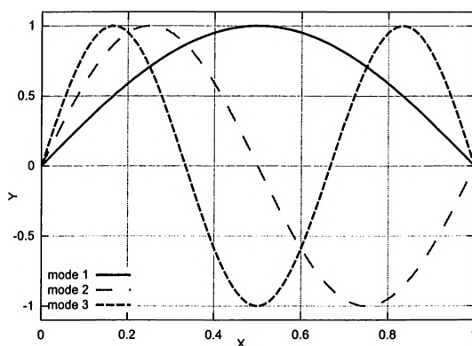
Figure 6.2 - Les 3 premiers modes de vibration de la poutre
