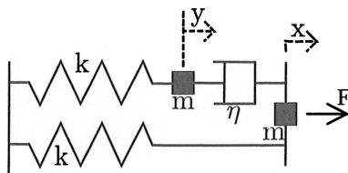
Figure 5.1 - Système masses-ressorts-amortisseur
