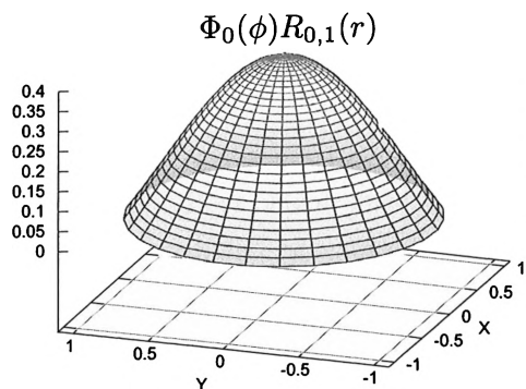
Figure 6.3 - Mode(0,1) du tambour
