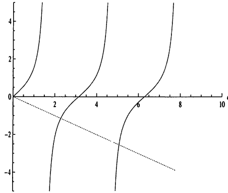
Figure 6.1 - Obtention graphique des \omega_n
