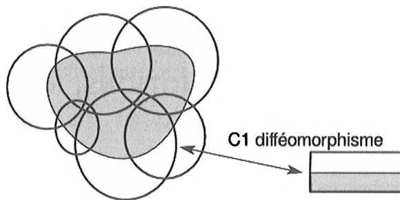
Figure D.1 - Cartes locales d'un ouvert
