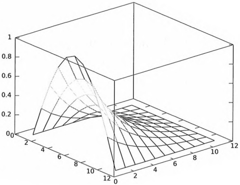
Figure 1.5 - Équation de Laplace
