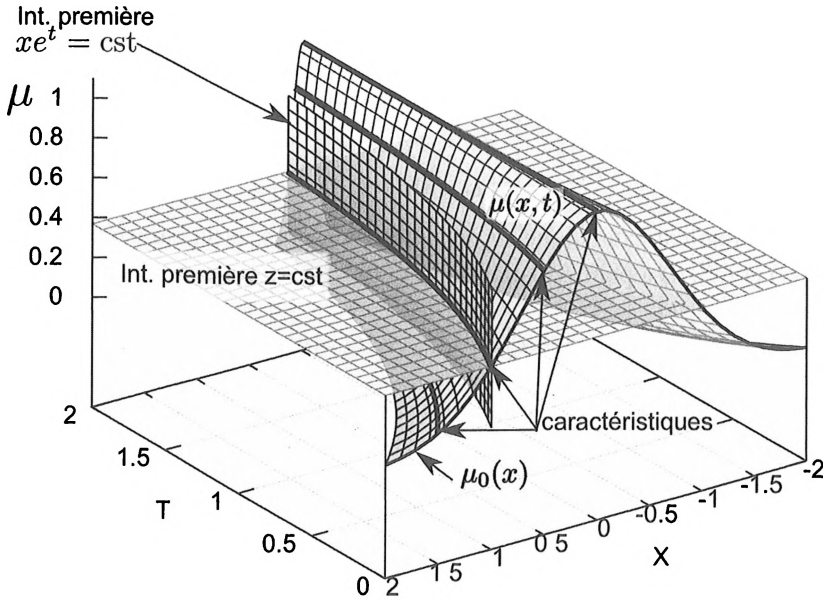
Figure 7.4 - Solution de l'équation du transport avec célérité variable
