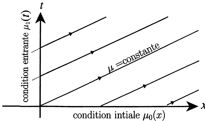
Figure 7.2 - Les caractéristiques de l'équation de transport de l'équation de transport dans le domaine x \geq 0 , dans le cas d'une célérité constante positive
