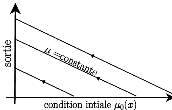
Figure 7.3 - Les caractéristiques de l'équation de transport de l'équation de transport dans le domaine x \geq 0 , dans le cas d'une célérité constante négative
