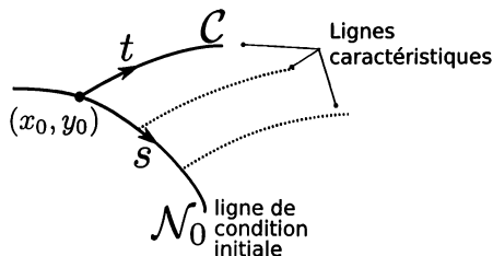
Figure 2.2 - Propagation de la donnée initiale le long de la caractéristique
