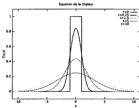
Figure 1.2 - Diffusion d'un créneau
