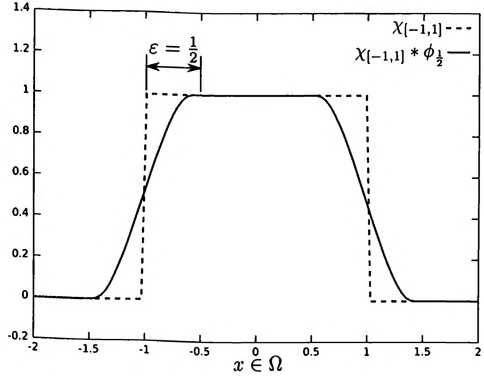
Figure 4.4 – Régularisation de l'indicatrice de [-1, 1]
