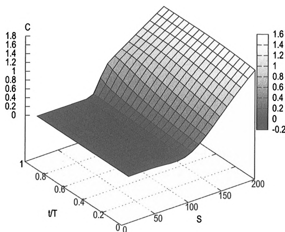
Figure 7.6 - Le « call », en fonction du prix du stock S et du temps t , pour E = 100 , r = 6\% , \sigma = 0.3 .
