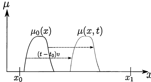
Figure 1.1 - Transport d'une répartition initiale
