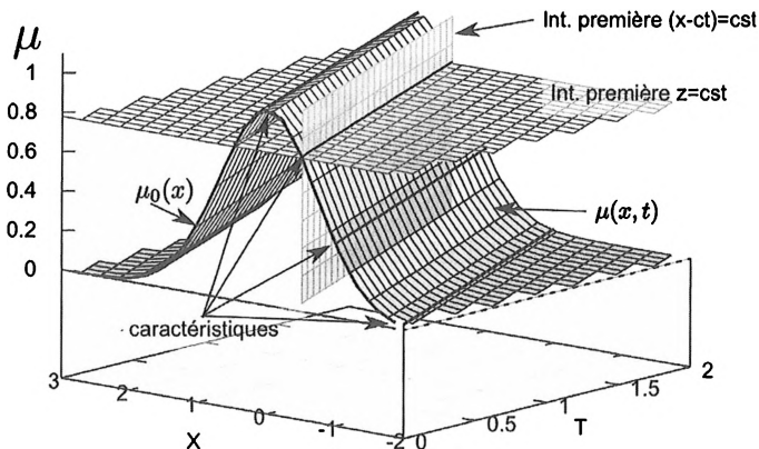
Figure 7.1- Solution de l'équation de transport avec célérité constante
