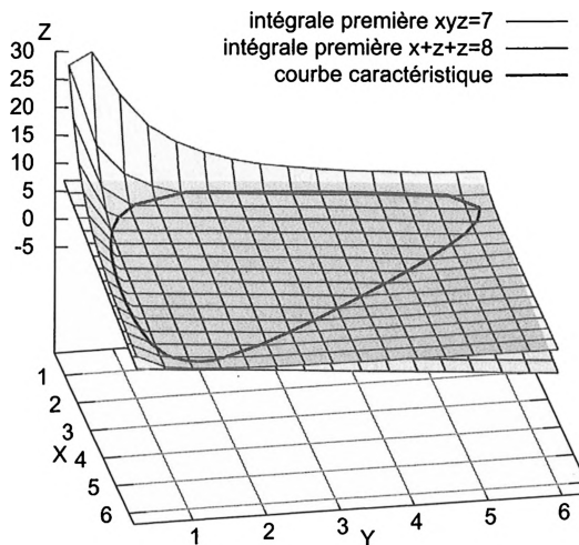
Figure 2.1- Intégrales premières indépendantes et courbe caractéristique sur le cadran x, y, z > 0 pour l'exemple 2.1
