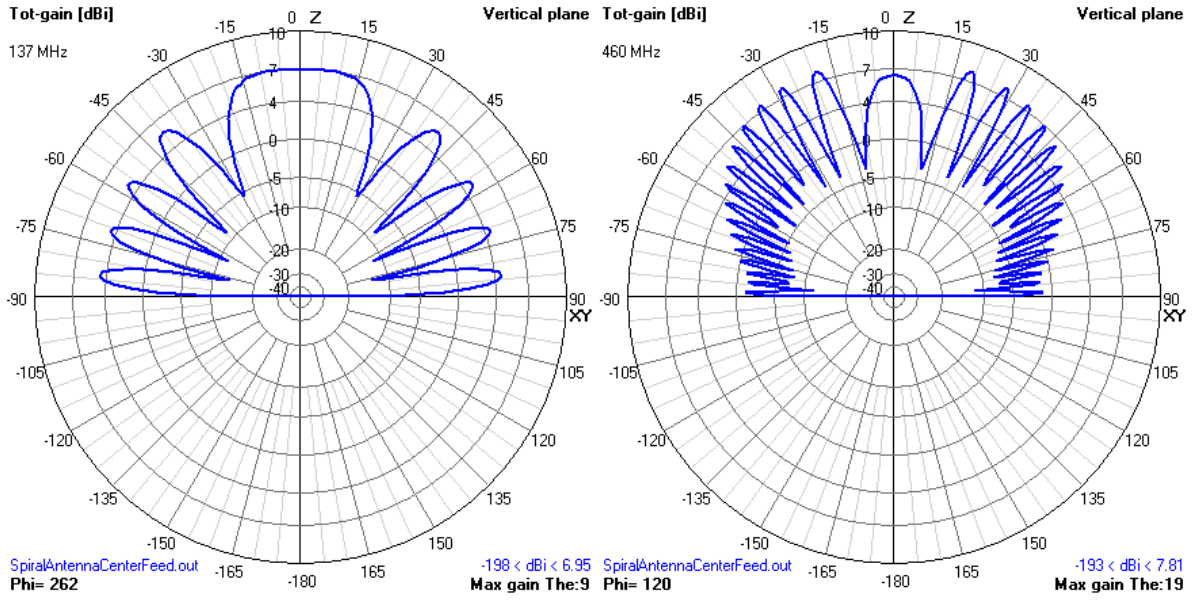
Left: 137 MHz. Right: 460 MHz.
