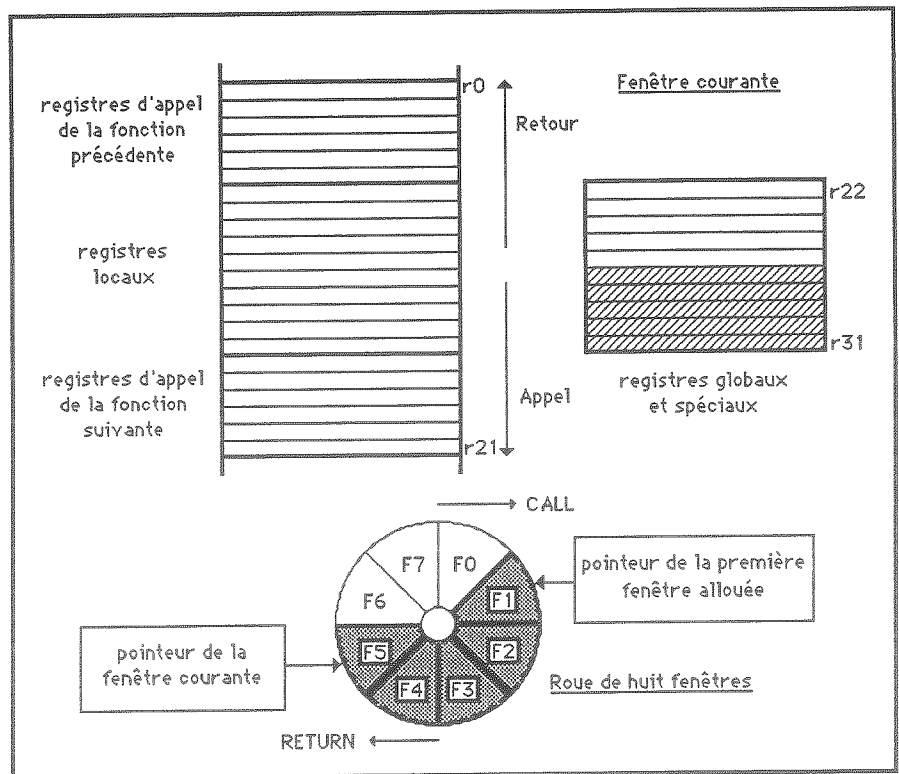
Fig. 31- Le mécanisme des fenêtres de registres
