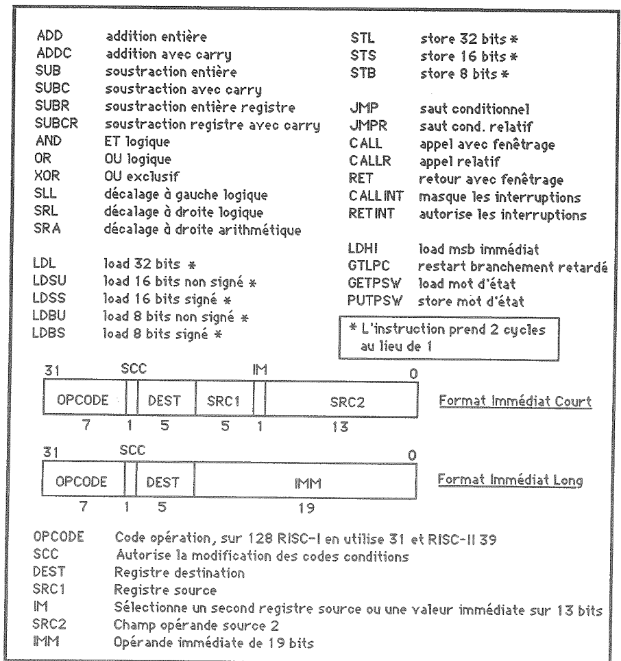
Fig. 8 - Le jeu d'instructions et les formats d'instructions RISC-I
