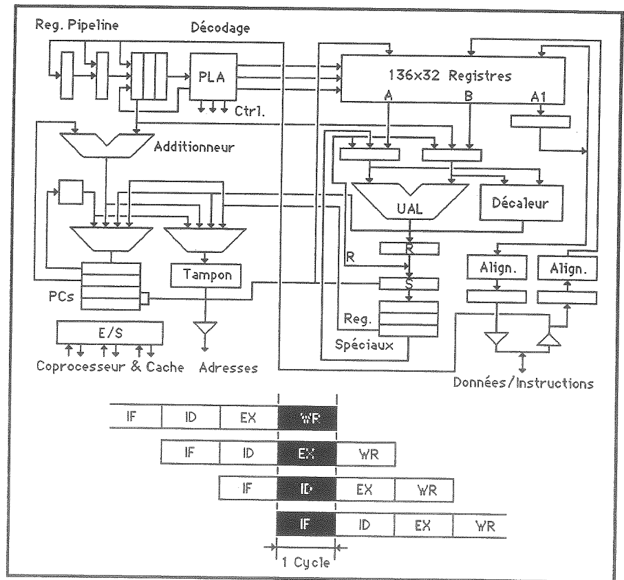
Fig. 36 - Synoptique et pipeline du processeur SPARC
