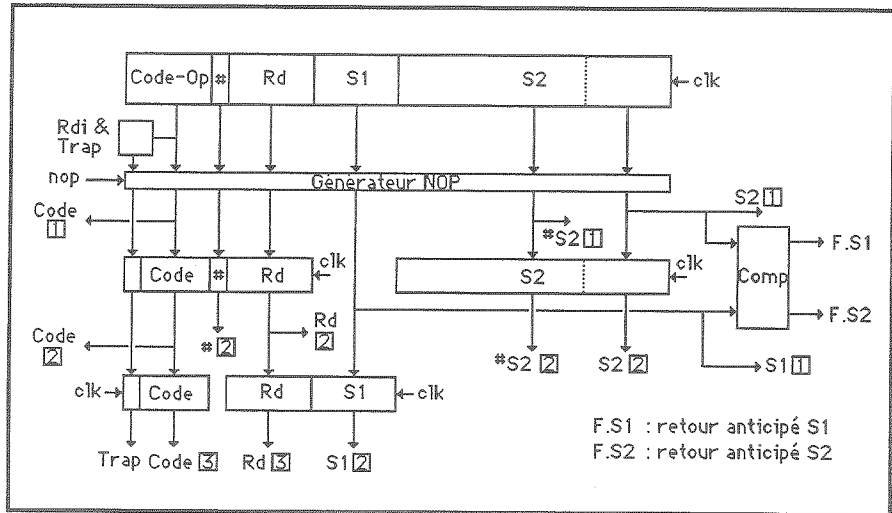
Fig. 75 - L'unité de séquençage et de décodage
