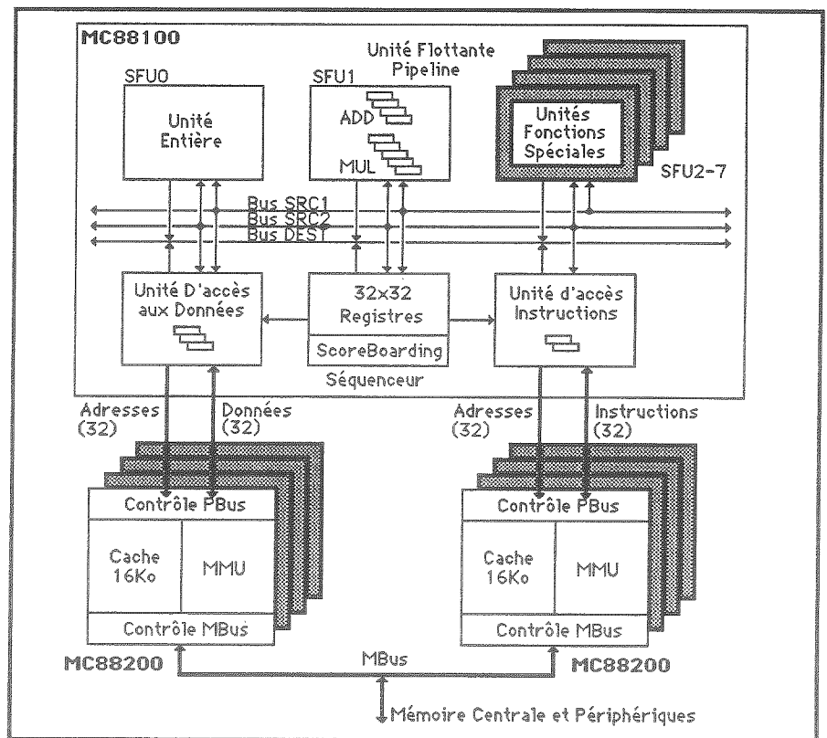
Fig. 43 - Synoptique du processeur MC88100
