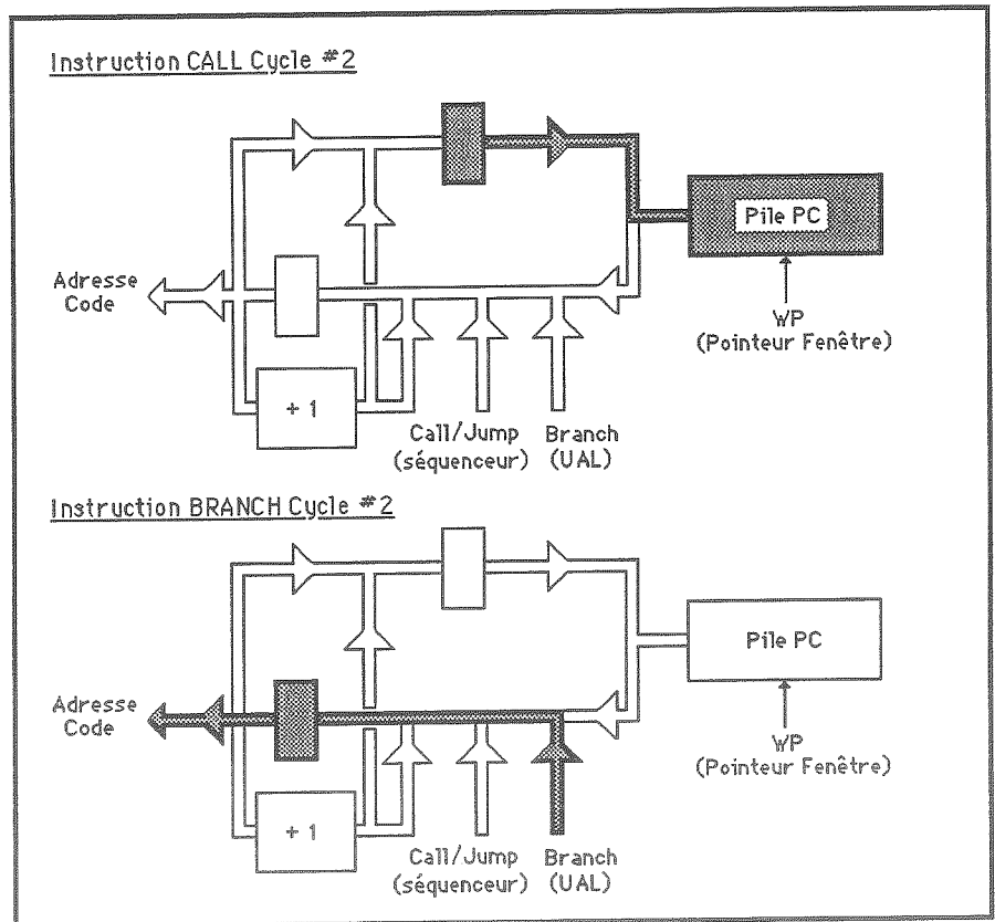
Fig. 82 - Séquencement du 2e cycle des instructions de branchement
